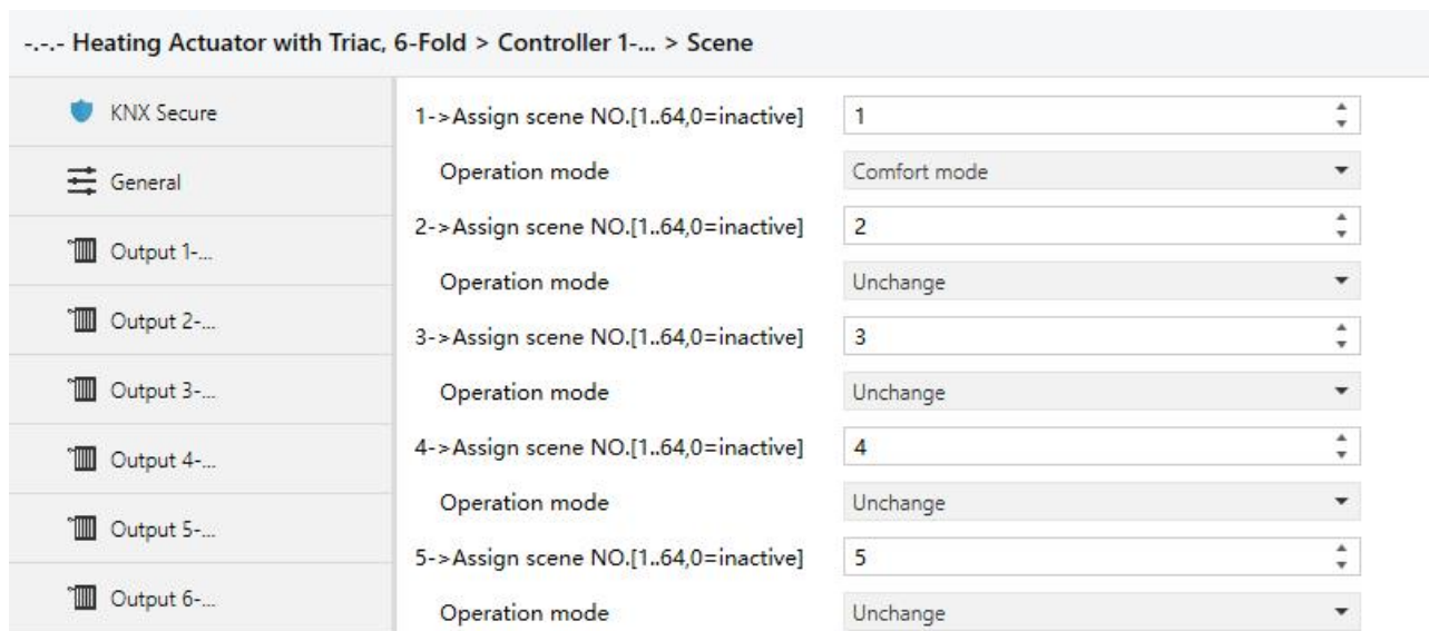
图 5.4.4 Scene” 参数设置界面
